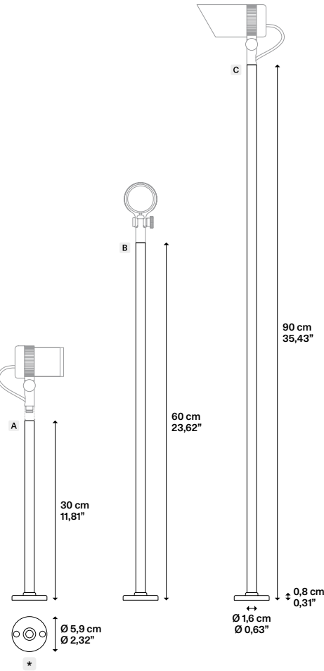
Stem with fixing base for surface installation Stelo con base di fissaggio per installazione a superficie
