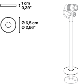
Cover for fixing base Copertura per base di fissaggio
