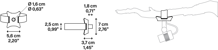
Fixing tree strap (max length 5 m – 196,85") Cinghia di fissaggio per albero (lunghezza max 5 m – 196,85")
