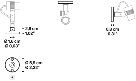
Fixing base Base di fissaggio
