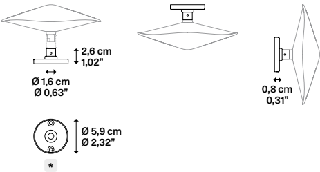
Fixing base Base di fissaggio
