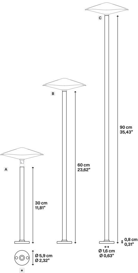
Stem with fixing base for surface installation Stelo con base di fissaggio per installazione a superficie
