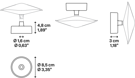
Stem with fixing base for surface installation Stelo con base di fissaggio per installazione a superficie
