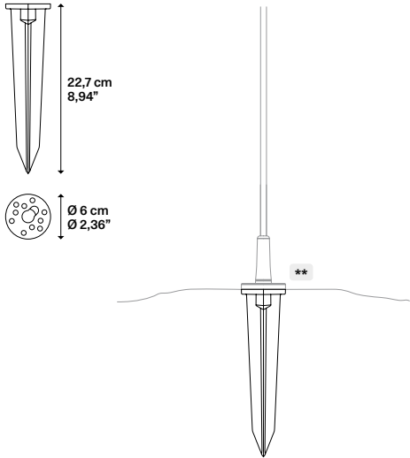
Spike for direct ground installation Picchetto per installazione nel terreno
