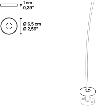
Cover for fixing base Copertura per base di fissaggio
